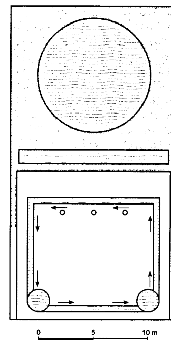
Erzwäscheanlage in Laureion (Grundriß).
